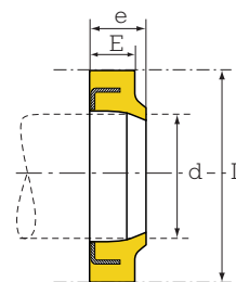
Type DRT
