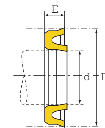
Type DRT
